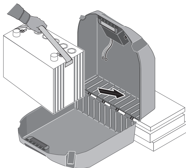
Figura 5: Instale la batería en la caja. Haga que alguien sostenga la caja mientras usted lo hace. Cuando la batería esté en la caja, conecte los conductores del cargador/control: +(Rojo) a +(Rojo), y -(Negro) a -(Negro).
