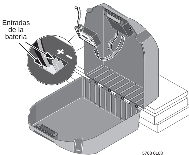
Figura 4: La entrada de la batería está dentro de la caja de la batería. Sostenga la caja cuando la abra. El sostén debe ser de un espesor mínimo de 4".
