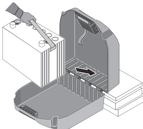
Figure 5 : Mettre la batterie dans son coffret. Demander à une autre personne de tenir le coffret pendant cette opération. Lorsque la batterie sera dans son coffret, brancher les fils du chargeur et du panneau de contrôle : + (Rouge) sur + (Rouge, et - (Noir) sur - (Noir).
