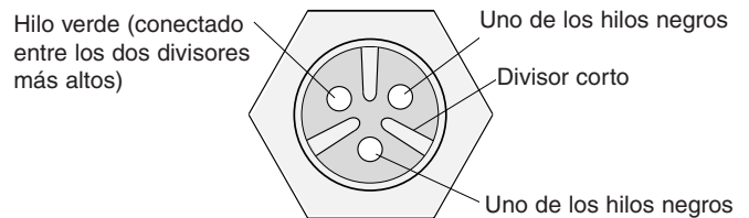
VISTA A-A
