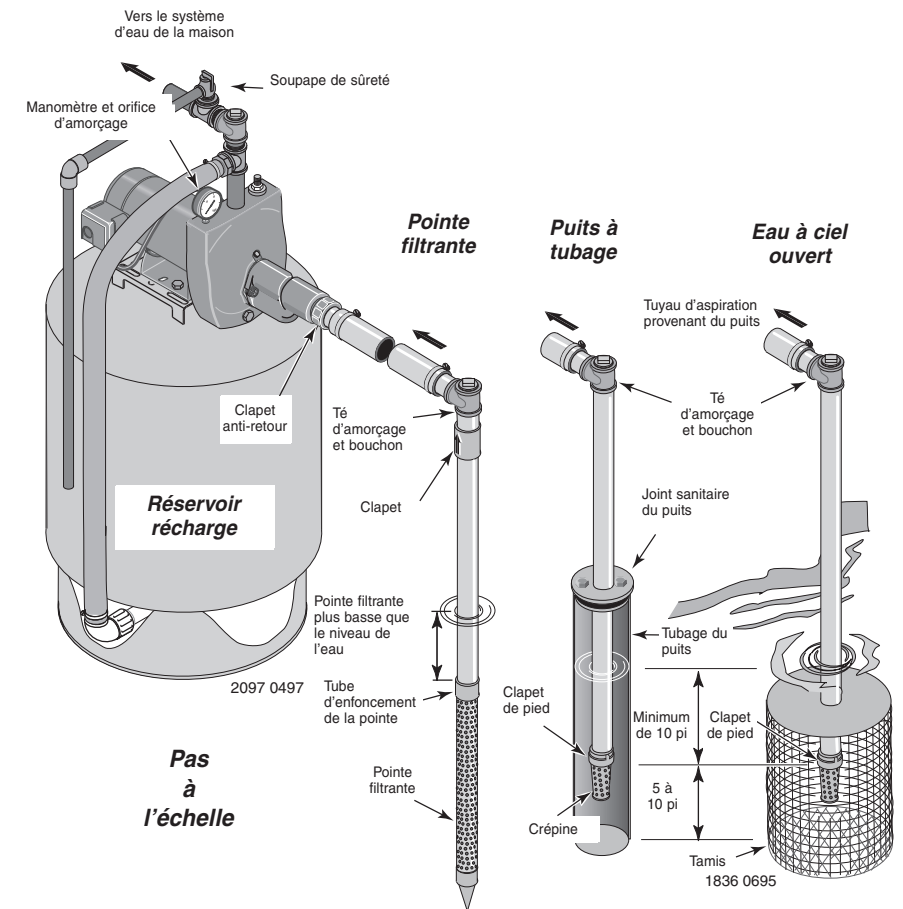
Figure 3 : Montage de l'éjecteur - puits peu profonds
