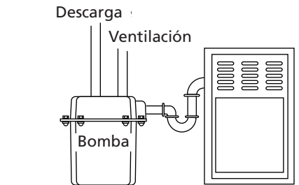
Figura 8 - Instalación típica para eliminar la condensación de acondicionadores de aire o el agua del deshumidificador
