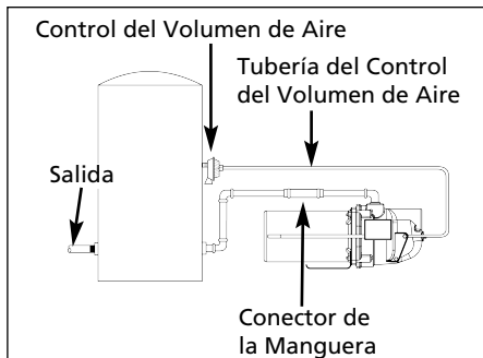
Figura 5 - Tanque Vertical
